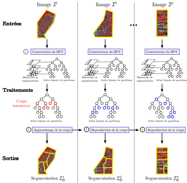
FIGURE 4: Approche de segmentation hiérarchique par BPT. En rouge : interactions de l'utilisateur. En bleu : traitements automatiques. En jaune : p imageries représentant p zones différentes mais centrées sur le même type d'objets d'intérêt.
