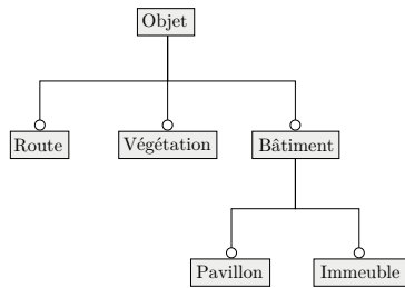
FIGURE 2: Exemple de hiérarchie de six concepts urbains.
