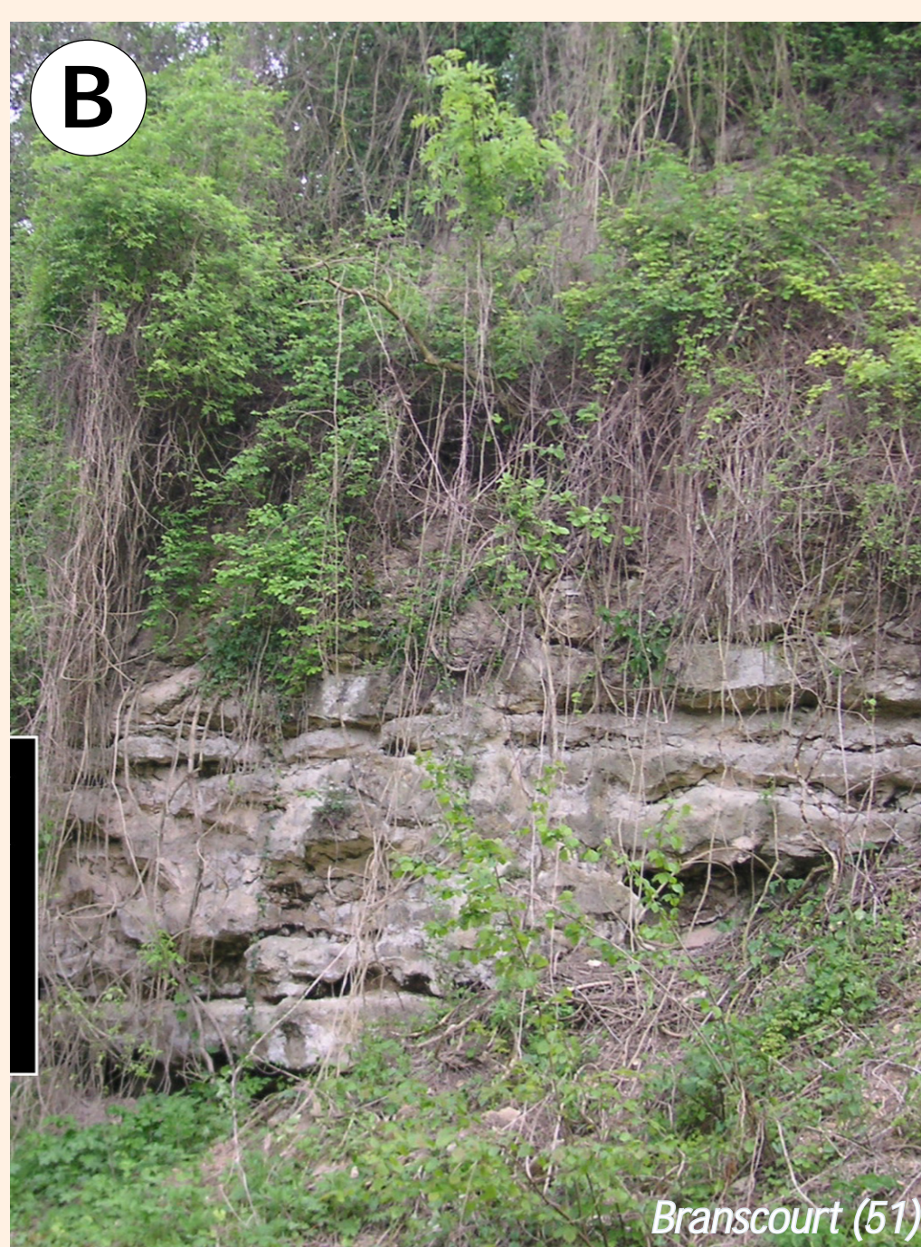
Exploités en souterrain dans la zone A, les calcaires à Ditrupe sont exploités à ciel ouvert dans la zone B. Et ce sont les bancs sous les calcaires à chailles qui sont exploités en souterrain.
