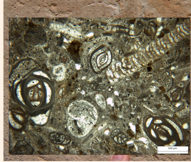
La principale pierre de taille des environs de Reims : un calcaire roux à millioles , Cardita et Orbitolites (Porosité 15 à 20 %)
