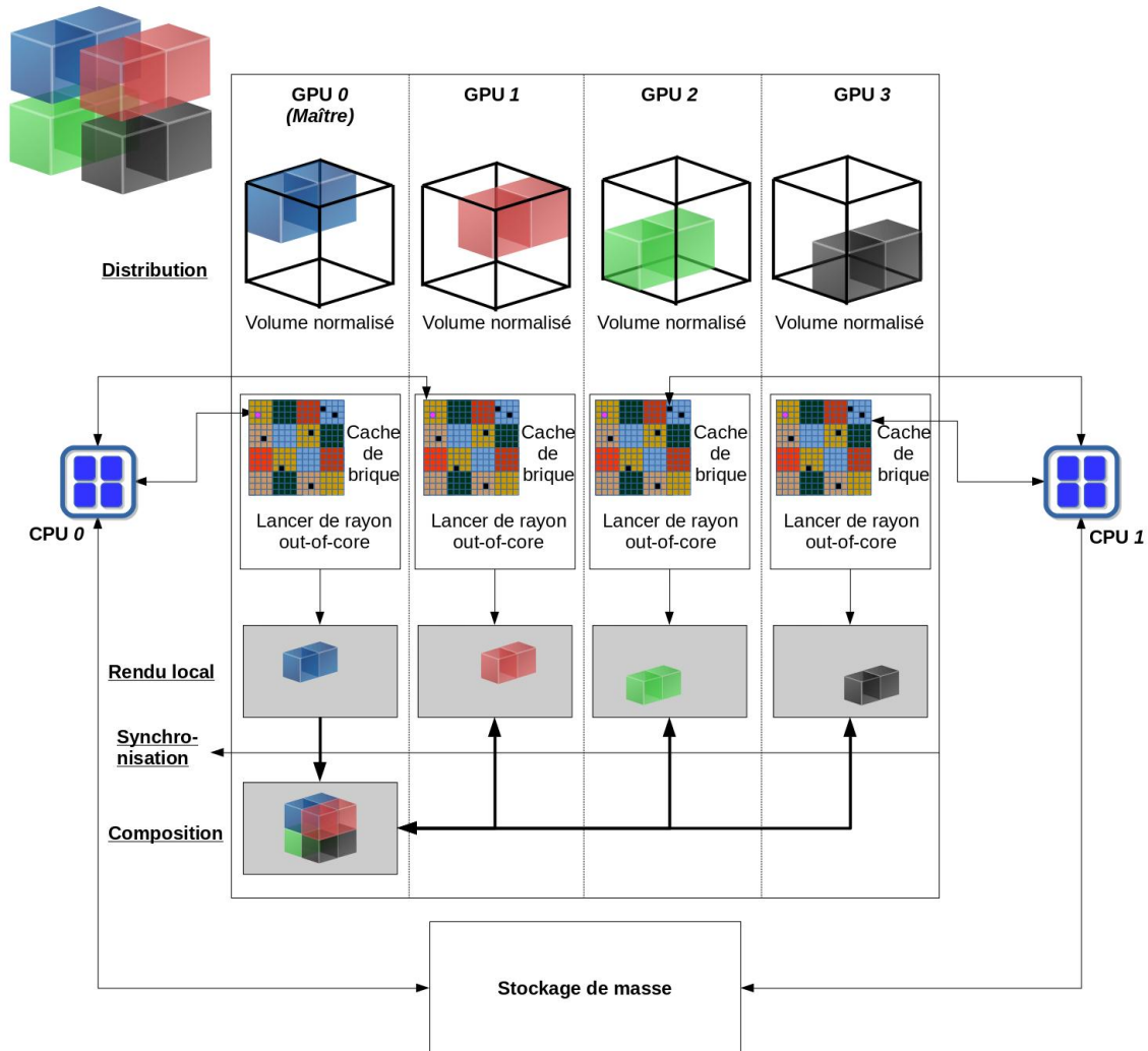
FIGURE 5.6 – Pipeline d'une approche "sort-last" de rendu volumique distribué out-of-core. Exemple de rendu distribué sur un système composé de quatre GPUs et de deux CPUs.
